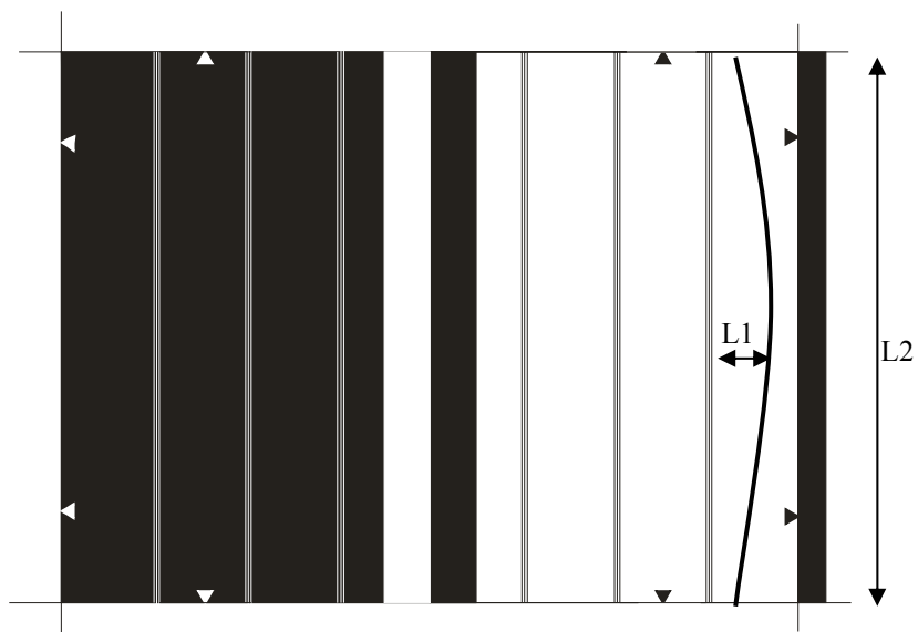
Рис. Г12 - Измерение линейных искажений
