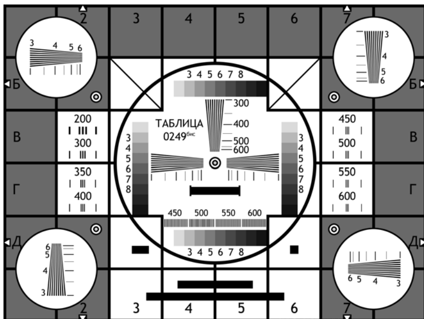
Рис. Б1 - Тестовая испытательная таблица «ТИТ-0249»
