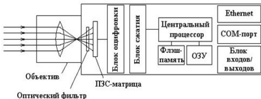
Рис. 10 - Устройство IP-камеры
