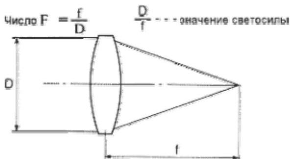
Рис. А3 - Светосила объектива
