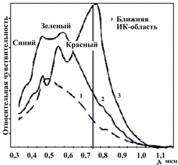
Рис. А2 - Спектральные характеристики чувствительности ПЗС: 1 – со строчным переносом, 2 – Exview ПЗС, 3 – ПЗС с кадровым переносом
