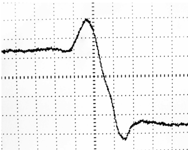
Рис. Г7- Реальные эюры напряжения от телекамеры в точке 5. (см. Рис. Г3)
