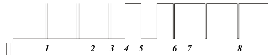
Рис. Г3 - Диаграммы напряжения (телевизионная строка) идеальной телекамеры от упрощенной тестовой таблицы
