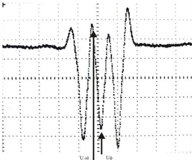
Рис. Г13 - Измерение контраста и глубины модуляции на фоне «белого» (см. Приложение А)
