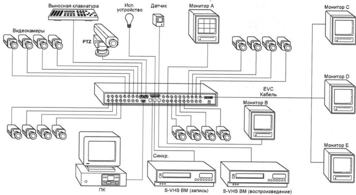
Рис.18 - Структура СОТ на базе универсального мультиплексора
