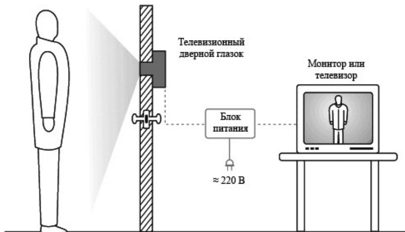
Рис. 15 - Структурная схема системы теленаблюдения на базе видеодомофона
