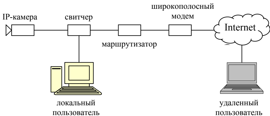
Рис.12 - Схема работы IP-камер с глобальных сетей
